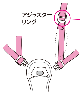
アジャスターリング 側面図
